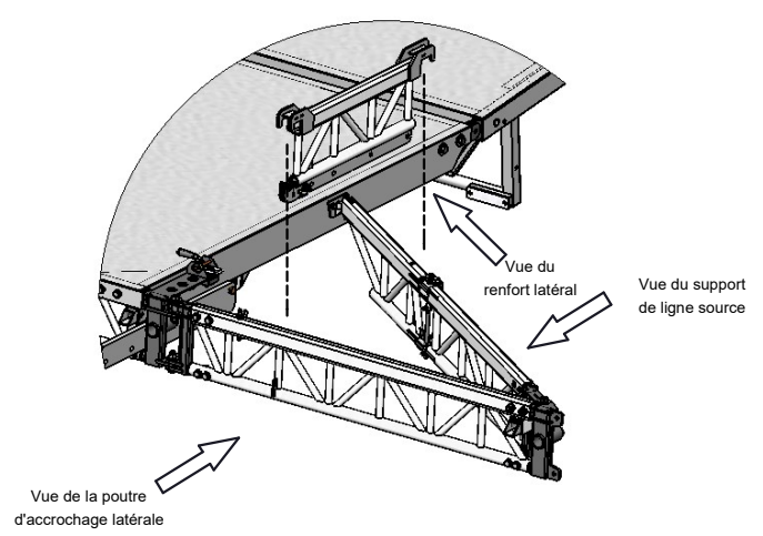
Structure avec support de ligne source
